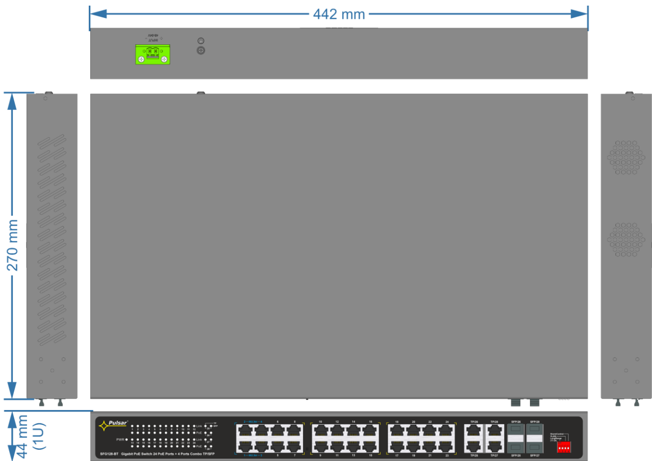
Rys. 4. Widok switch'a.
