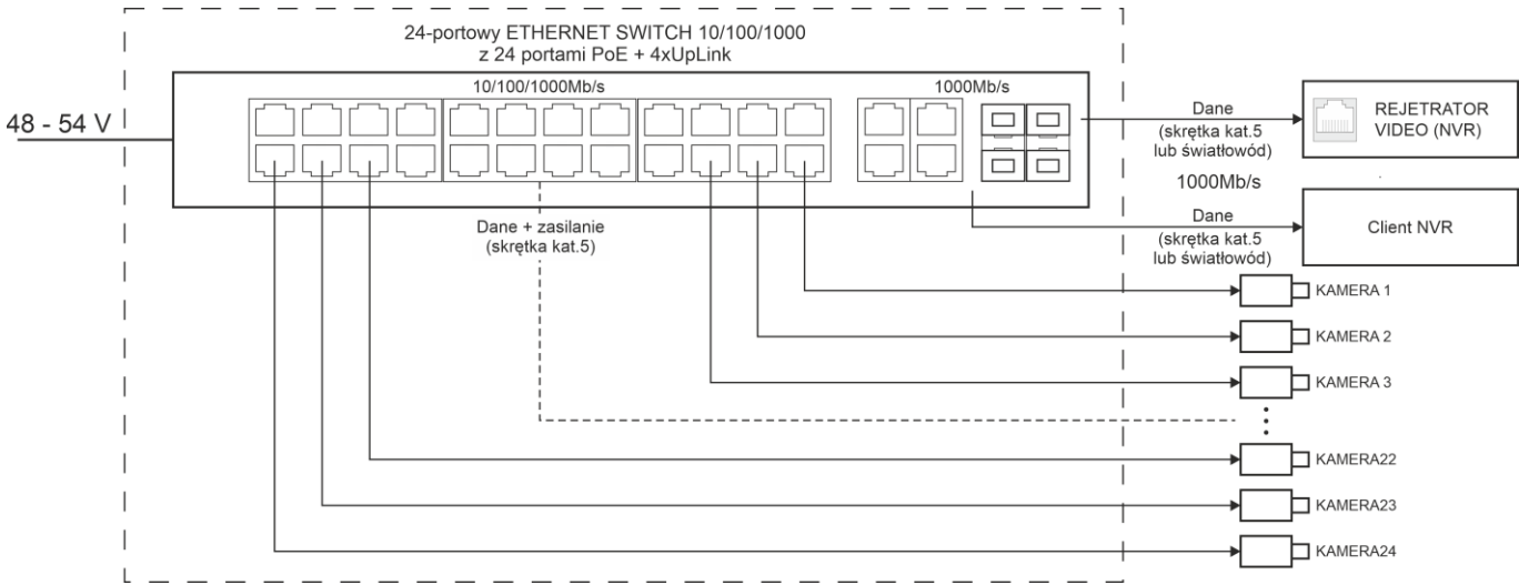
Rys. 1. Schemat blokowy.
