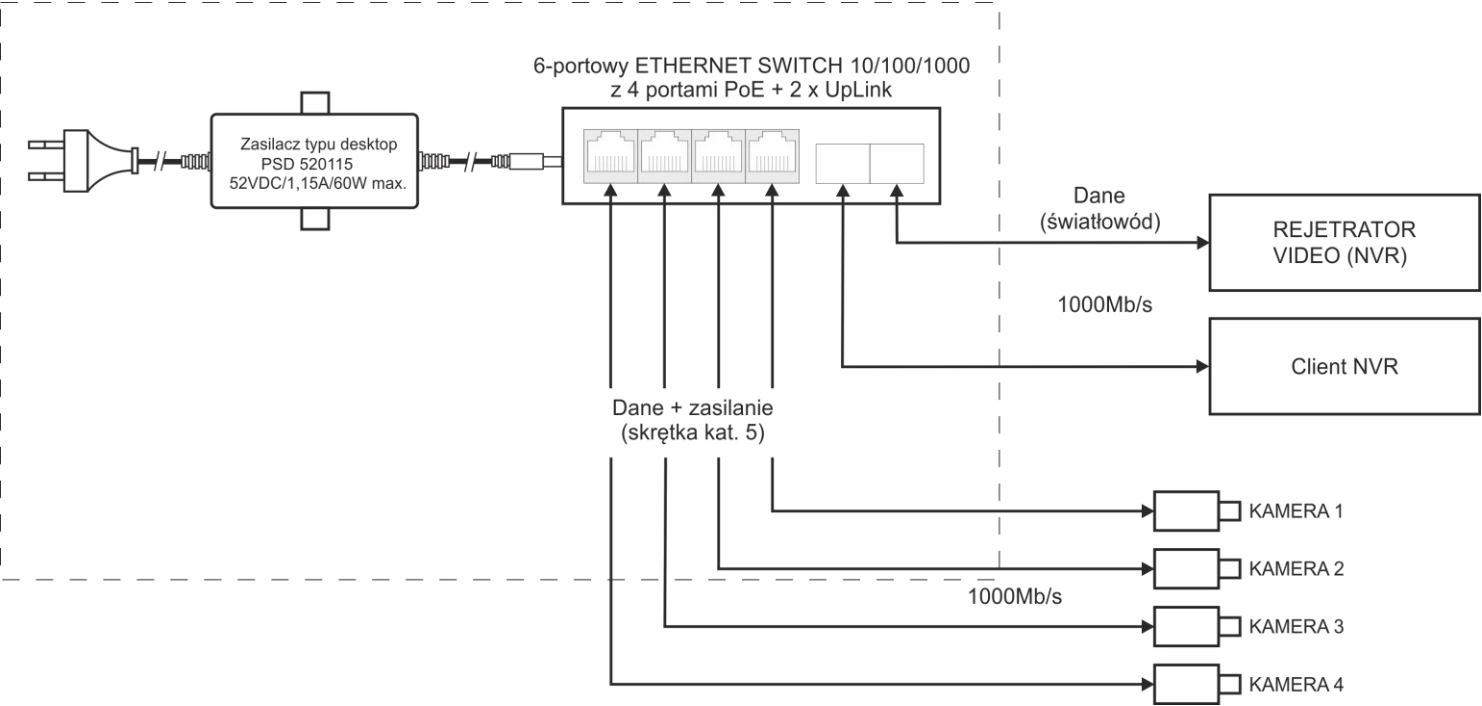
Rys. 1. Schemat blokowy.
