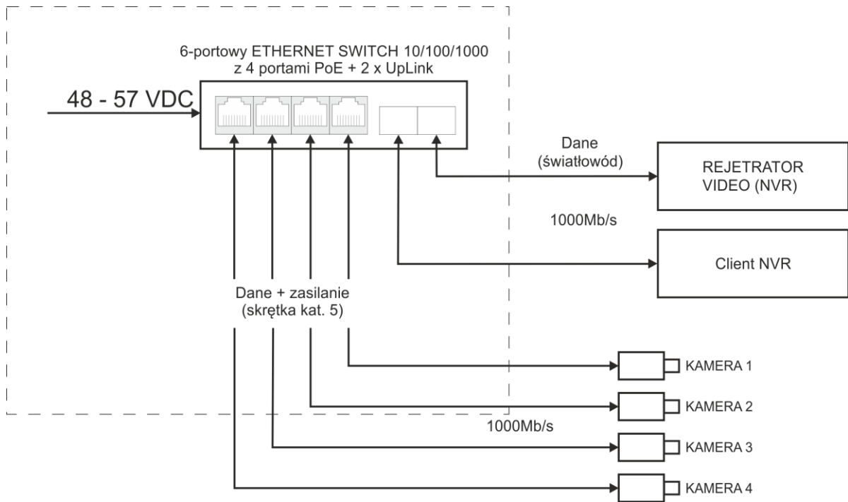
Rys. 1. Schemat blokowy.
