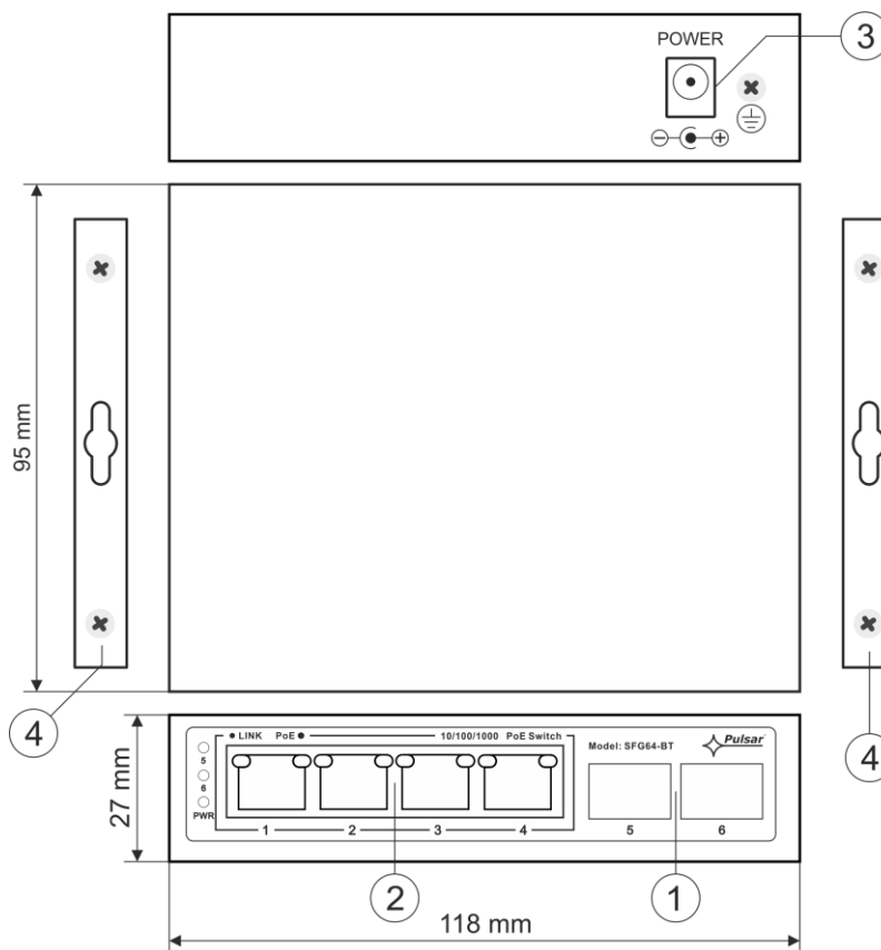
Rys. 2. Widok switch'a.
