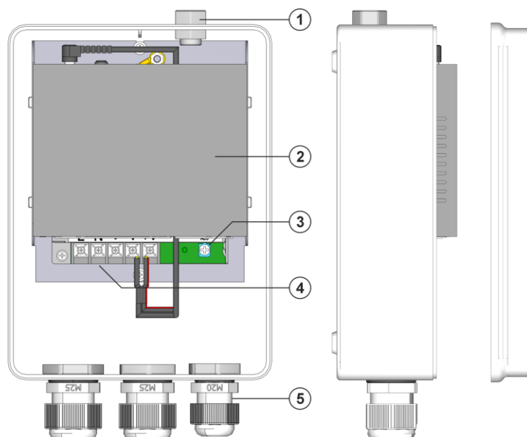
Rys. 2. Widok obudowy.
