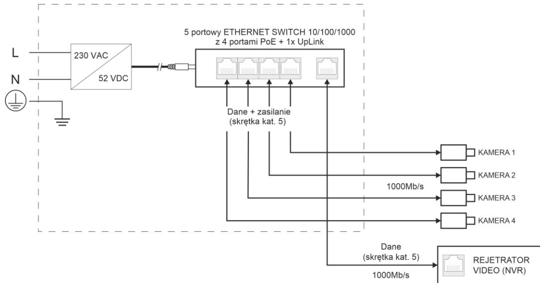
Rys. 1. Schemat blokowy.
