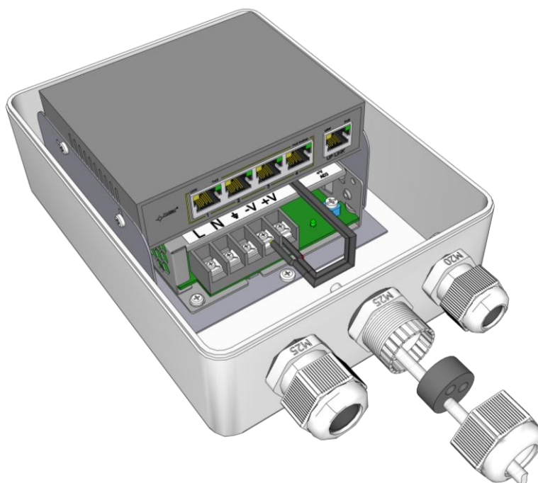
Rys.4. Przykład sposobu montażu urządzenia.
