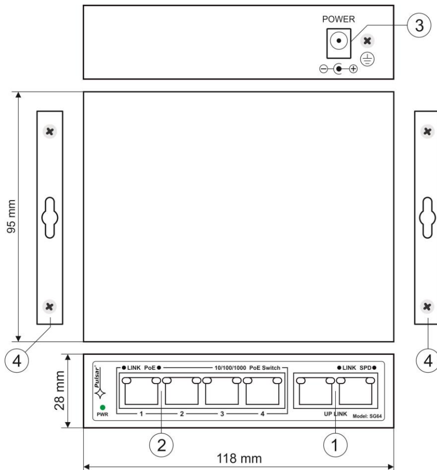
Rys. 2. Widok switch'a.
