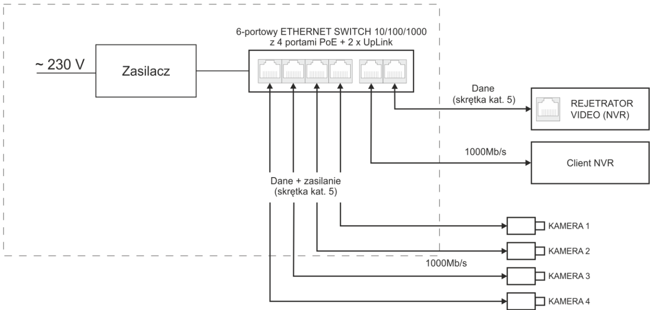
Rys. 1. Schemat blokowy.
