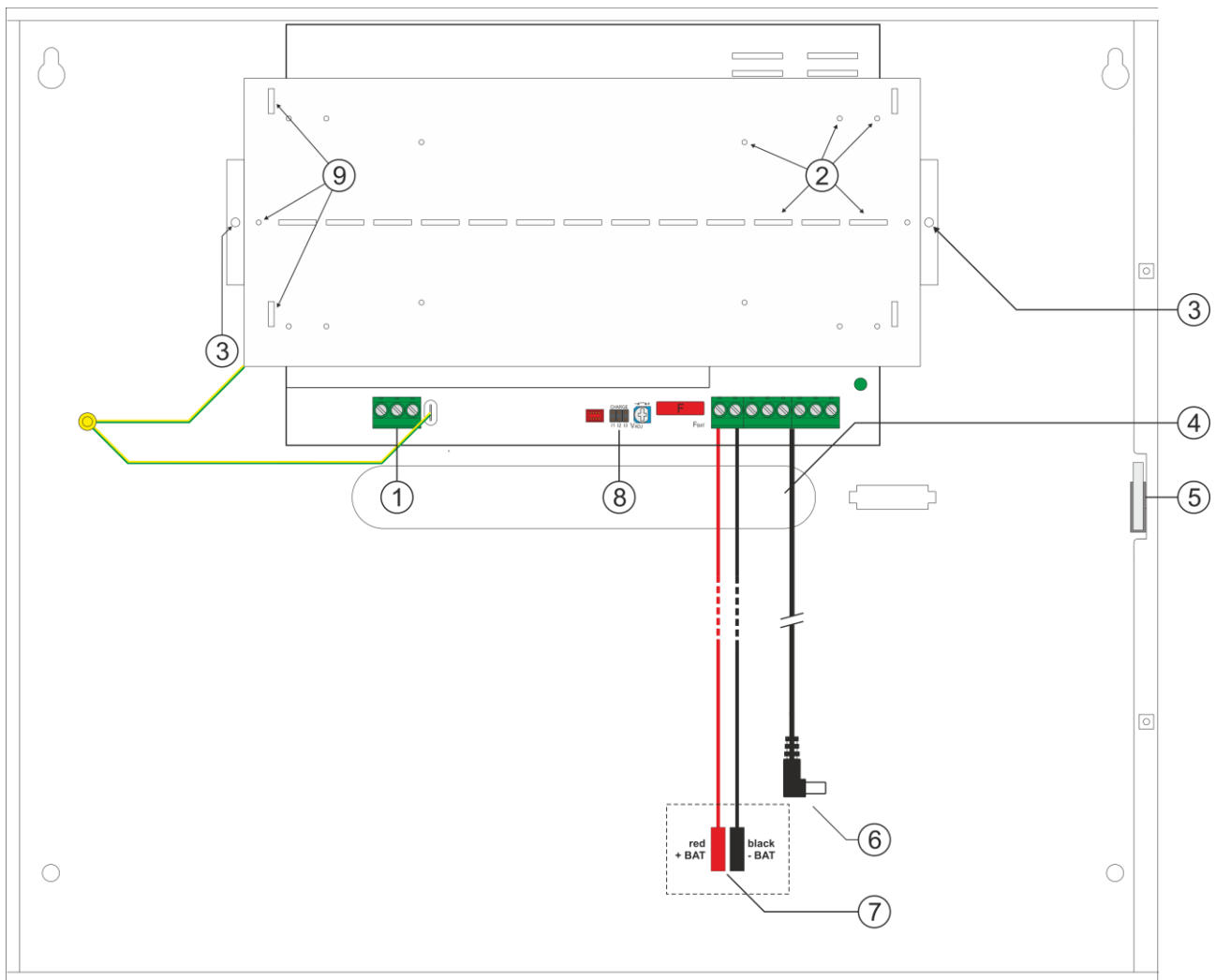
Rys.3. Widok zasilacza.
