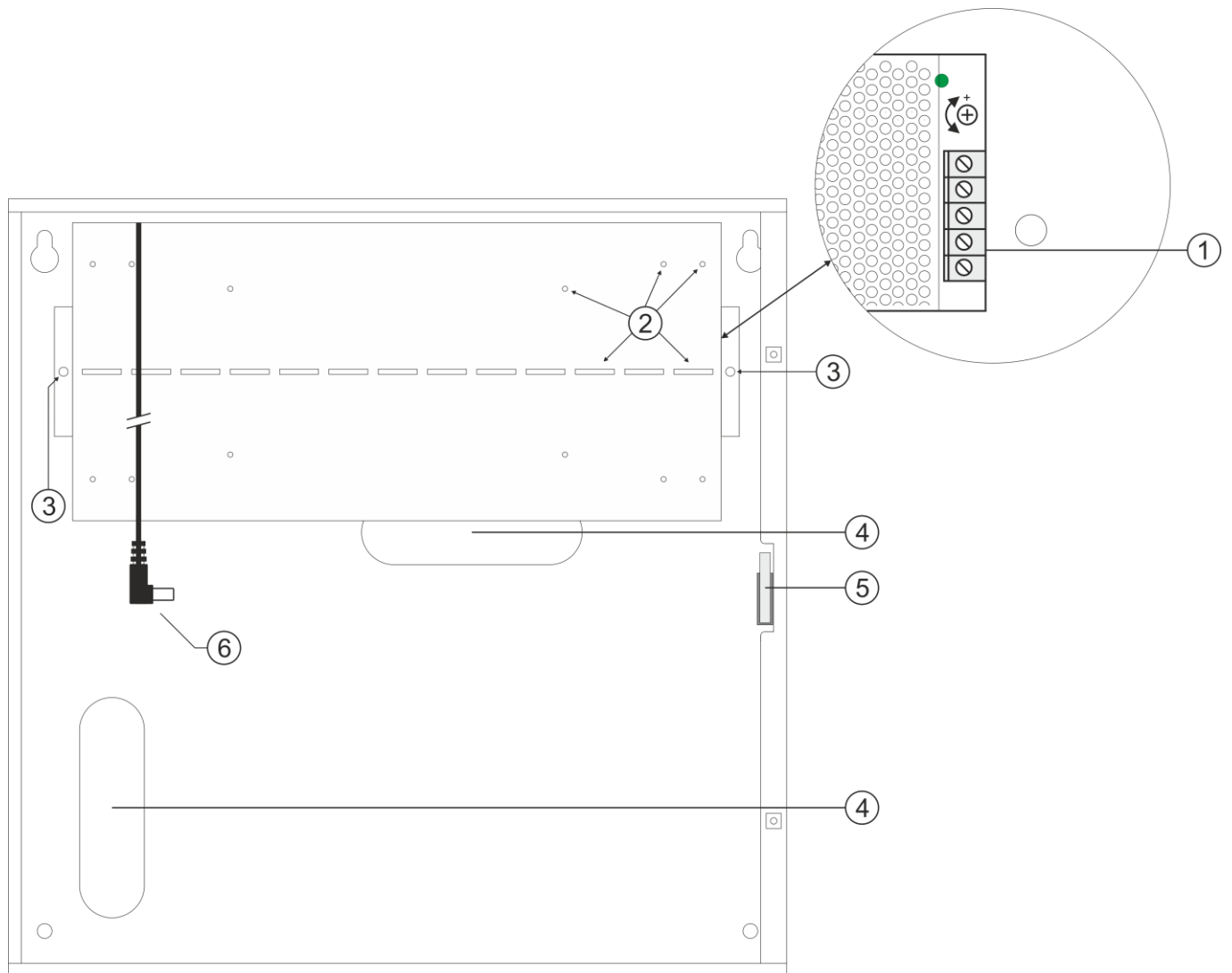
Rys.3. Widok zasilacza.
