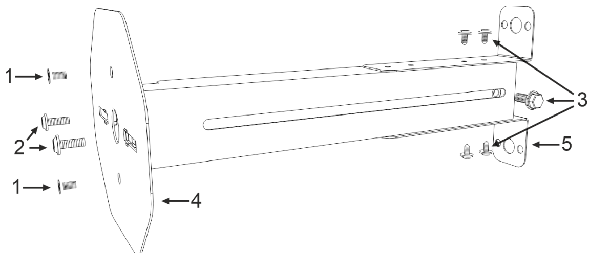
Rys.2. Montaż uchwyty
