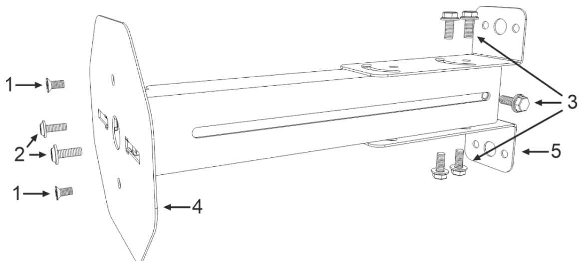
Rys.2. Montaż uchwyty
