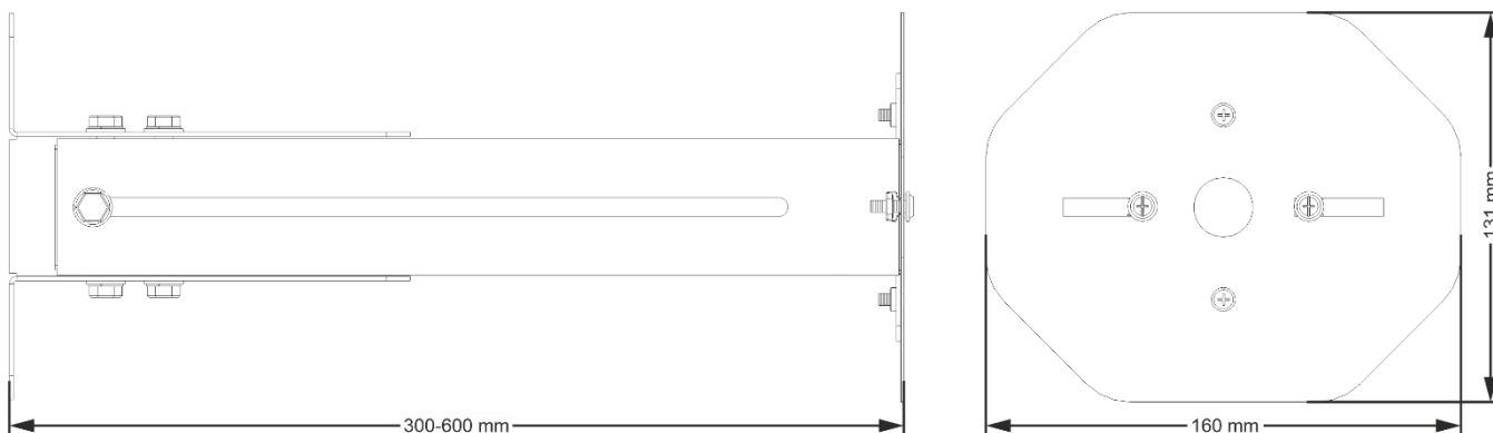
Rys.1. Wymiary
