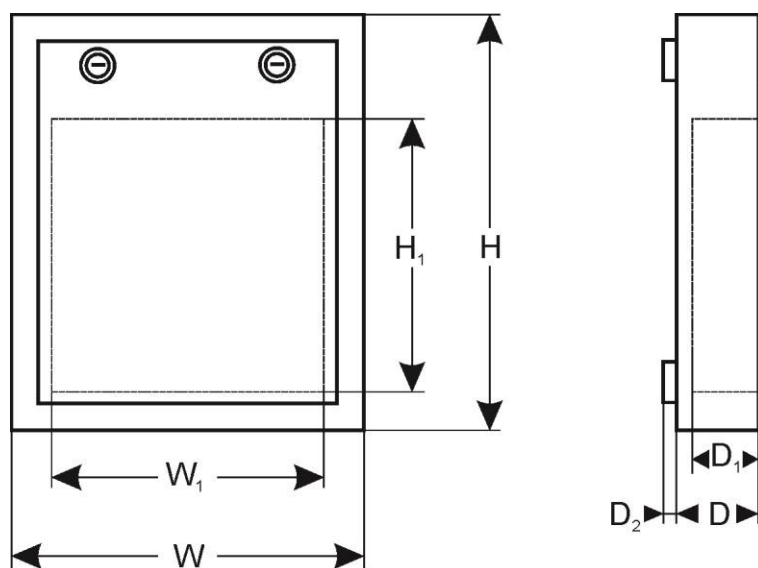
Obrázok 1. Rozmery.
