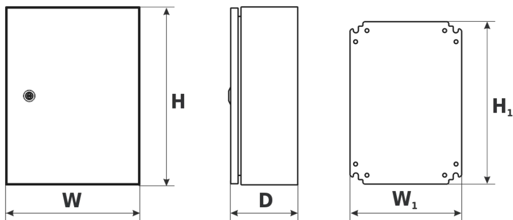
Obr. 2. Rozmery.
