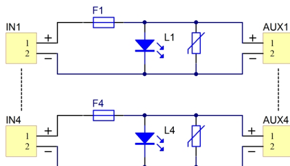
Obr. 2. Elektrická schéma.
