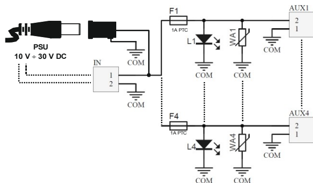
Rys.2. Elektrická schéma.
