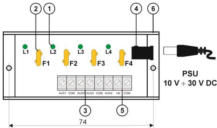
Obr. 1. Náčrt modulu.
