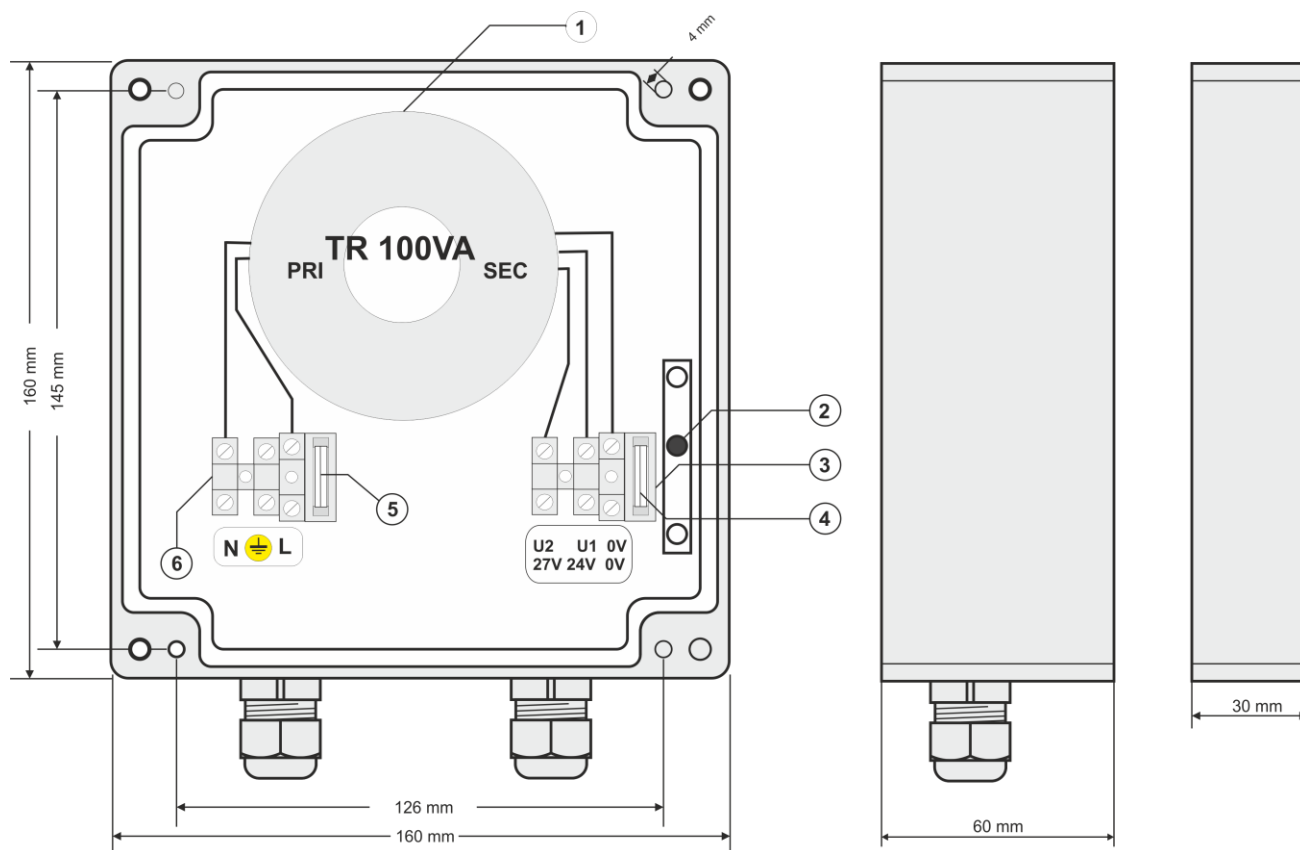
Obr.2. Rozmery zdroja.
