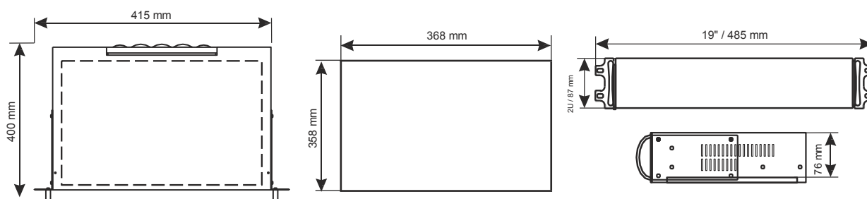
Montáž na lištu ARAS600N/800N/1000N
