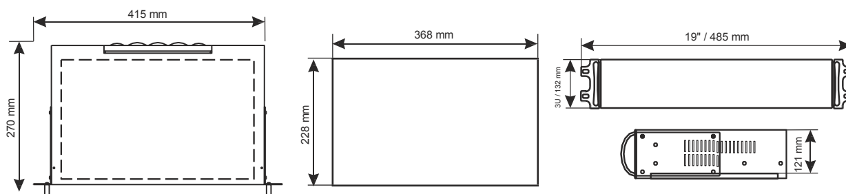
Montáž na lištu ARAS450N
