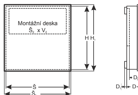
Nástěnná konstrukce
