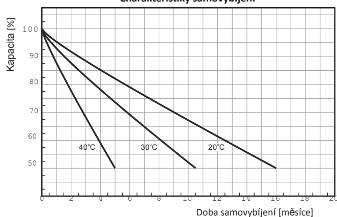
Charakteristiky samovybití
