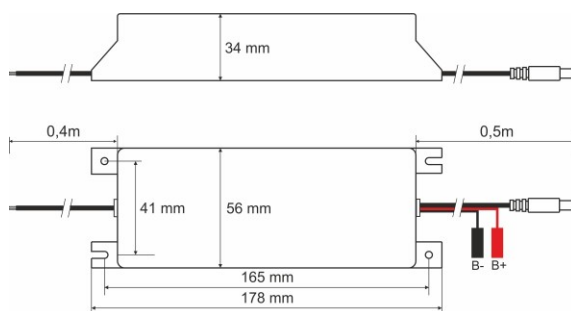
Obr.1 Rozměry napájecího zdroje.
