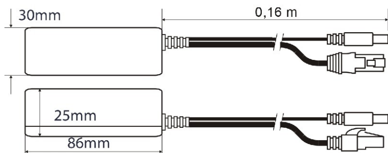
Obr. 1. Mechanický pohled.
