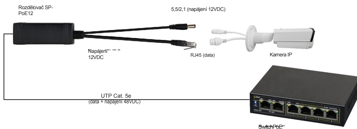
Obr. 2. Příklad propojení se switchem PoE.
