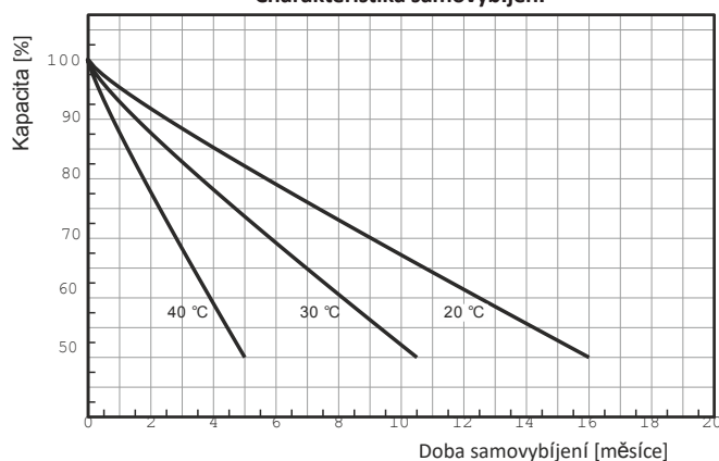
Charakteristika samovybíjení
