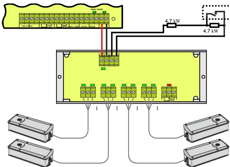
Beispiel für den Anschluss des sequenziellen Moduls EN54C-LS4.
