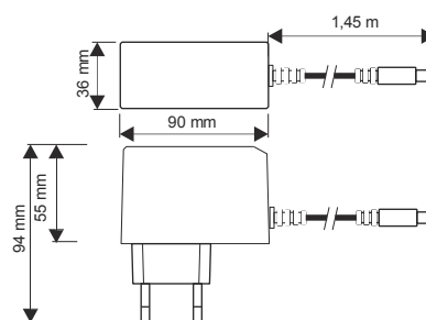
Abb. 1 Abmessungen des Netzteils.
