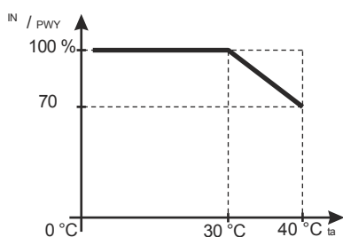
Grafik 1. Zusammenhang zwischen Ausgangsstrom und Umgebungstemperatur.
