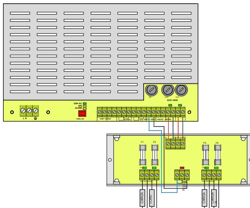
Ejemplo de conexión con módulo de fusibles EN54C-LB4.
