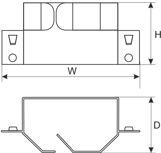
Lado derecho del armario RACK
