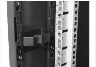
Lado izquierdo del armario RACK
