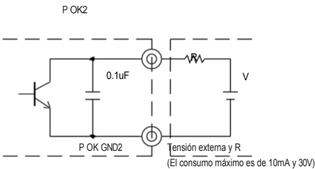
Fig. 4.3 Circuito interno de P OK2 (Método de colector abierto)
