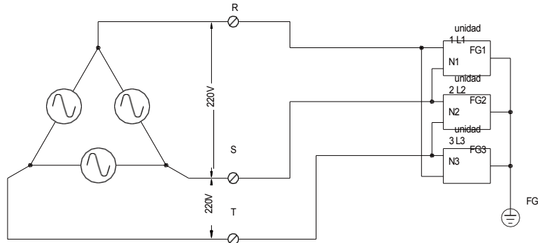
FIG. A: SISTEMA 3 \psi 3W 220VAC
