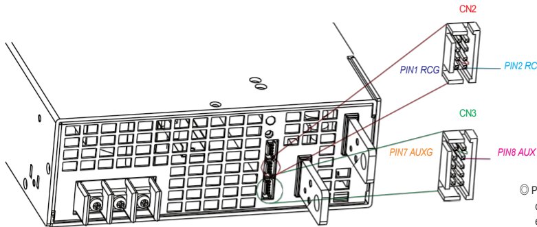
Ejemplo 3.2(A): Utilización de una fuente de tensión externa
