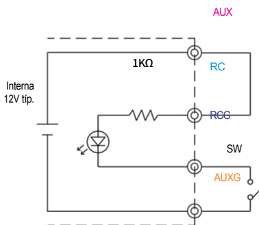
Ejemplo 3.2(C): Utilización de la salida auxiliar interna de 12V
