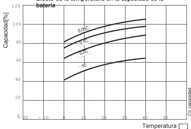
Efecto de la temperatura en la capacidad de la batería
