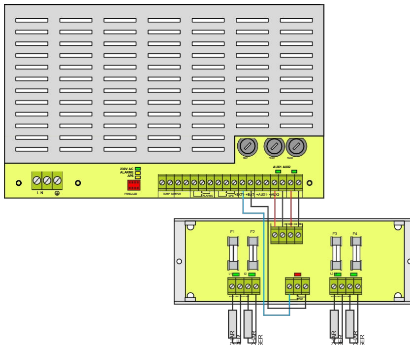
Exemple de connexion avec le module de fusibles EN54C-LB4.
