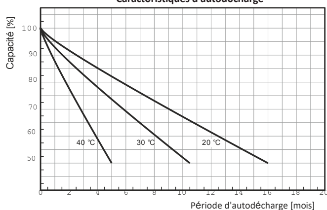
Caractéristiques d'autodécharge
