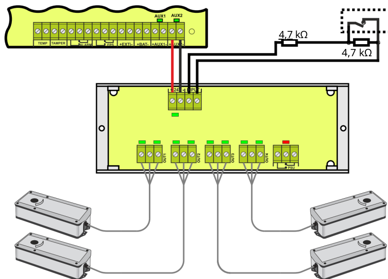
Παράδειγμα σύνδεσης της μονάδας διαδοχικής ενεργοποίησης EN54C-LS4.
