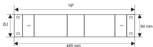
Πίσω όψη του ντουλαπιού RACK της σειράς RS/ZRS
