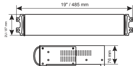
Szerelés ARAS600N/800N/1000N sínen
