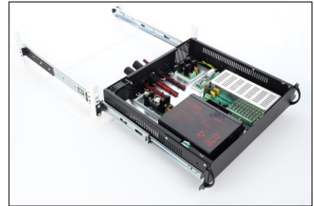
Szerelés ARAS600N/800N/1000N sínen
