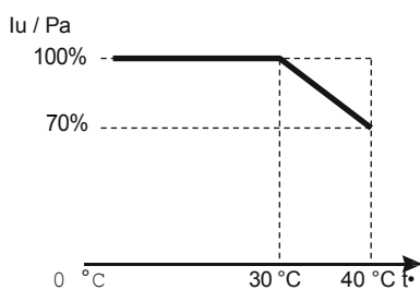
1. ábra. A kimeneti áram és a környezeti hőmérséklet közötti összefüggés (pillanatnyi terhelés).
