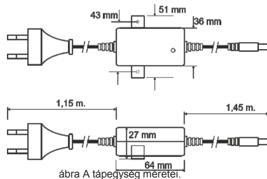
ábra A tápegység méretei.
