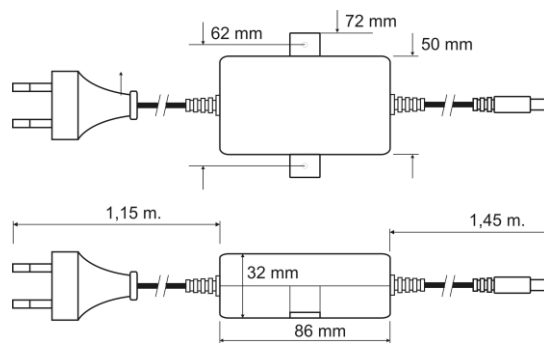
1. ábra: A tápegység méretei.
