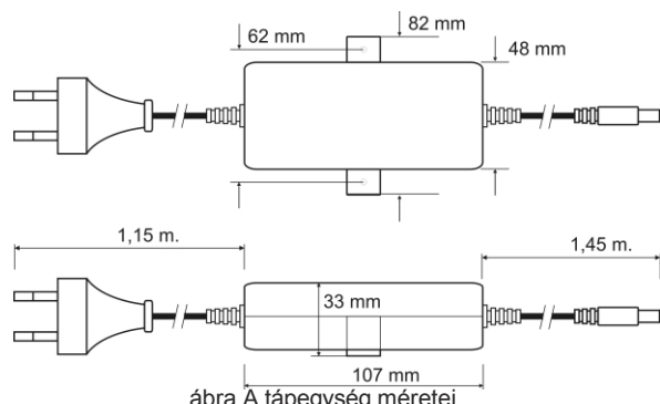
ábra A tápegység méretei.
