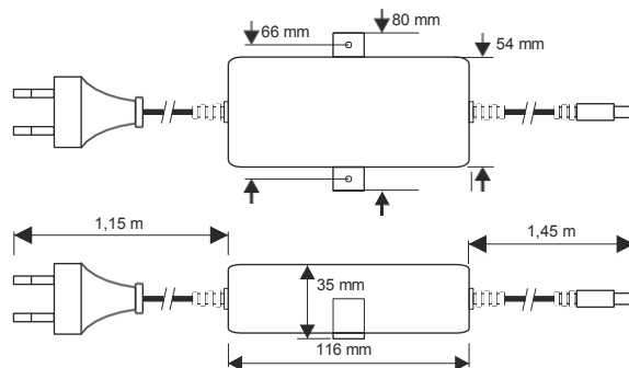
1. ábra A tápegység méretei.
