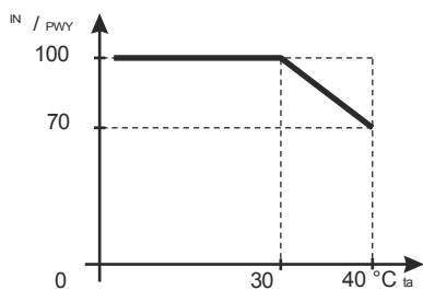
1. ábra A kimeneti áram és a környezeti hőmérséklet közötti kapcsolat (pillanatnyi terhelés).
