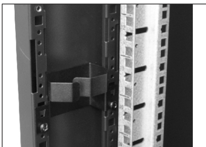
A RACK szekrény bal oldala
