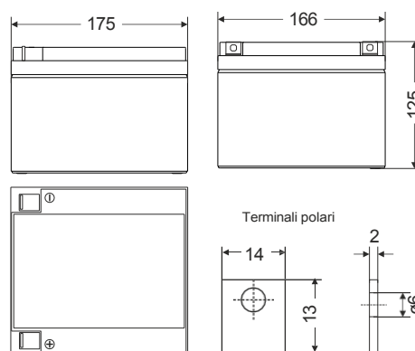
Dimensioni [mm] Tolleranza: +/- 2 mm;
