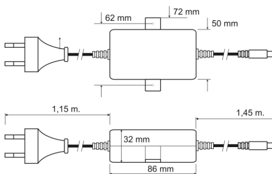
Fig. 1 Dimensioni dell'alimentatore.
