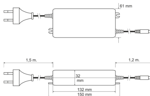
Fig. 1. Dimensioni dell'alimentatore.
