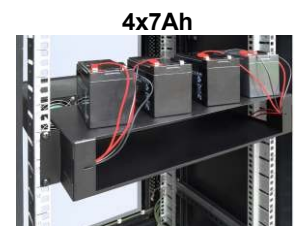
Vista posteriore dell'armadio RACK della serie RS/ZRS
