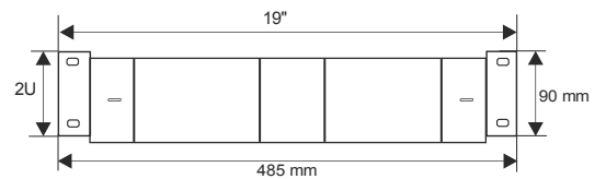
Vista posteriore dell'armadio RACK della serie RS/ZRS
