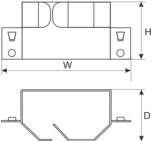
Lato destro dell'armadio RACK
