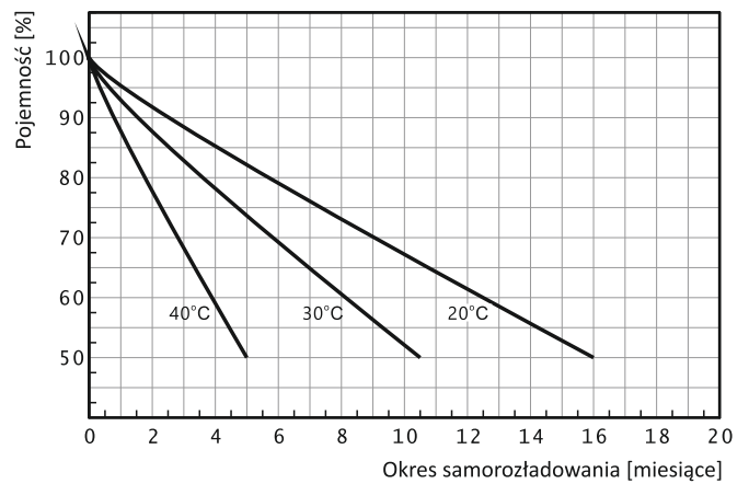
Charakterystyki samorozładowania
