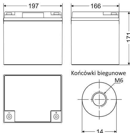
Wymiary w [mm] Tolerancja: +/- 2mm;
