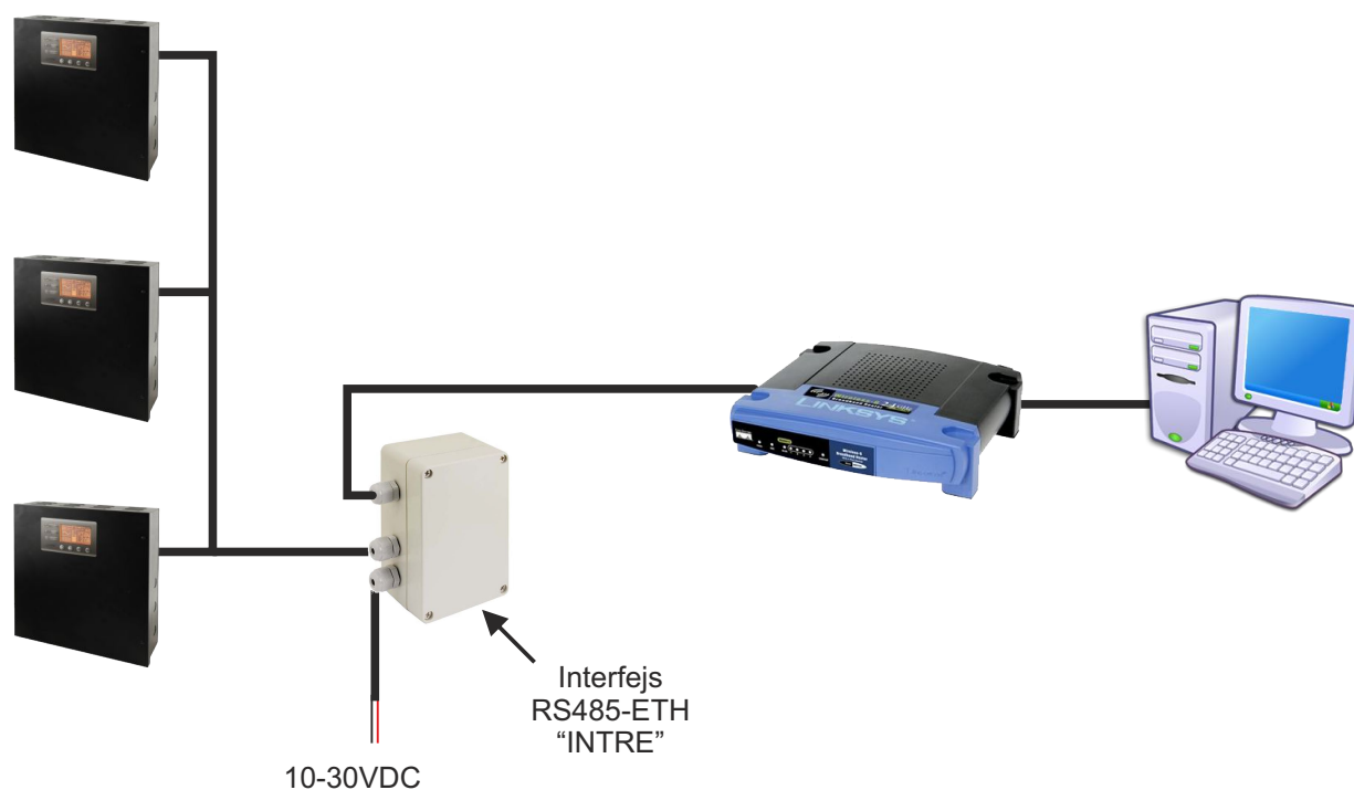
Komunikacja Ethernet z wykorzystaniem interfejsu RS485-Ethernet.
