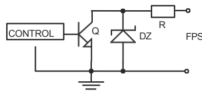
Elektrická schéma výstupu OC.
