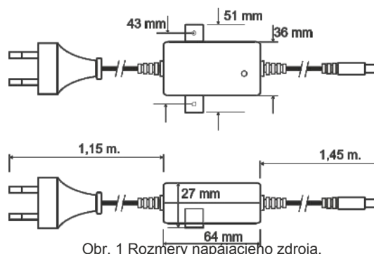
Obr. 1 Rozmery napájacieho zdroja.
