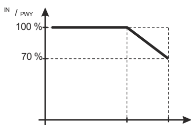
Graf 1. Vzťah medzi výstupným prúdom a okolitá teplota (okamžité zaťaženie).
