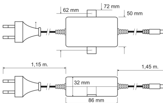
Obr. 1 Rozmery napájacieho zdroja.
